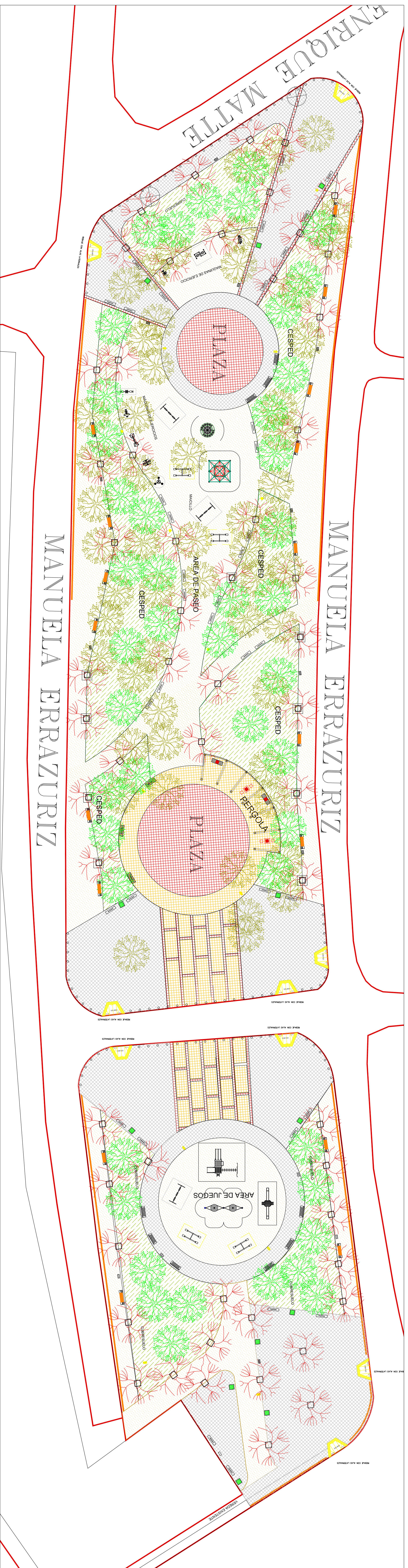
EMPLAZAMIENTO ESCALA 1:2000
